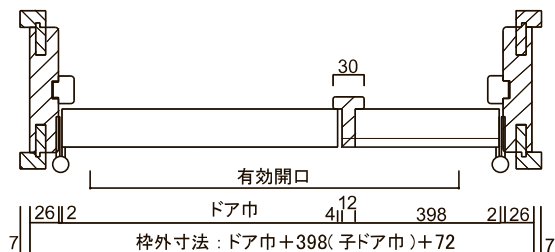
横断面図(親子ドア)
