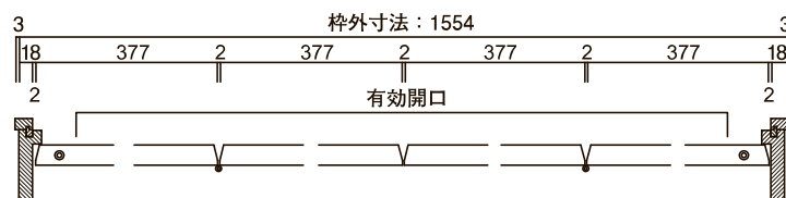
4枚扉 横断面図
