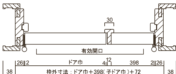
横断面図(親子ドア)
