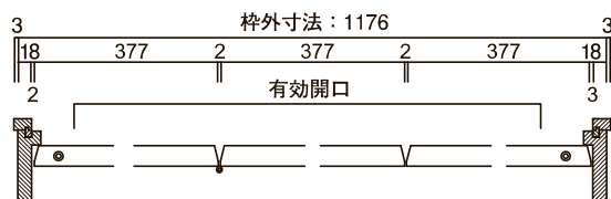
3枚扉 横断面図
