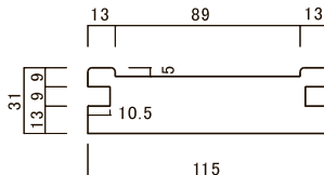
縦枠(引違い用)
