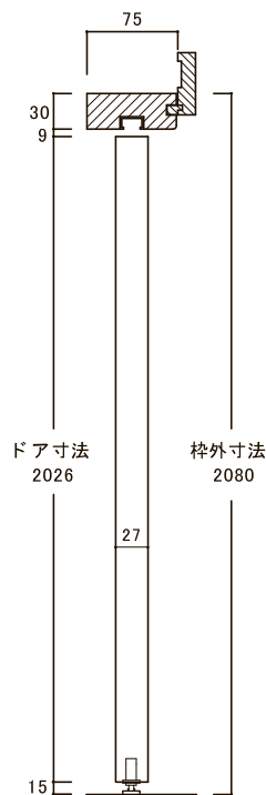
縦断面図
