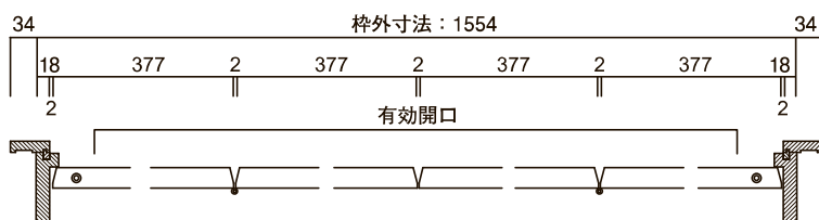
4枚扉 横断面図
