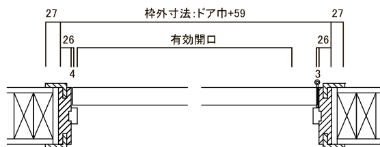
横断面図
