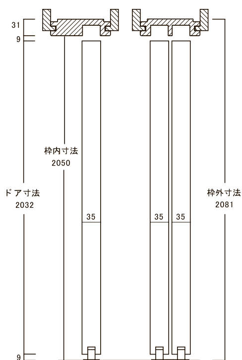
縦断面図
