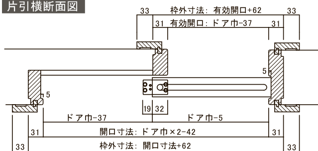
片引横断面図
