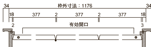
3枚扉 横断面図
