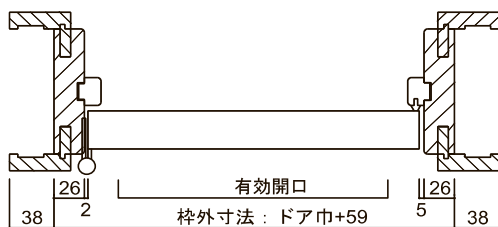
横断面図(親子ドア)
