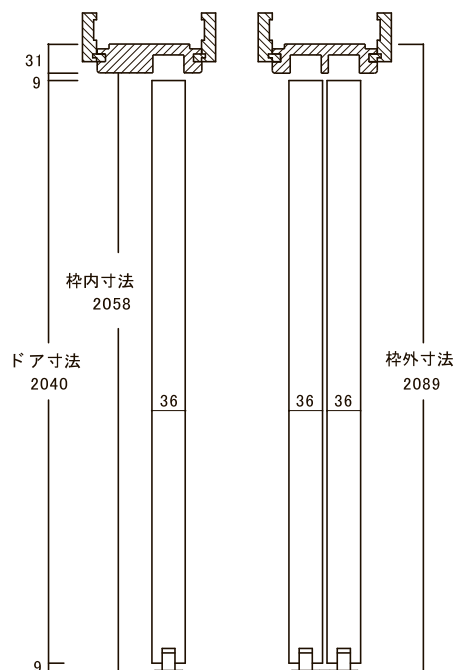
縦断面図
