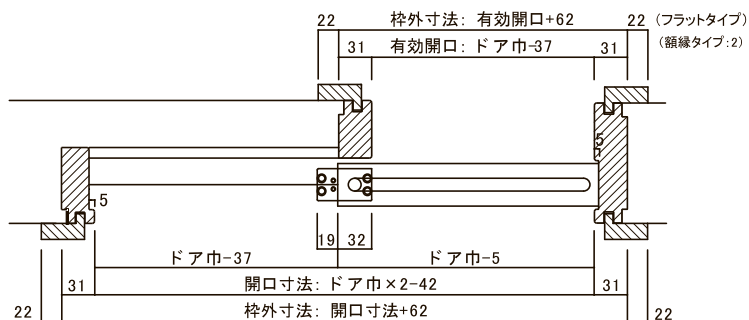
片引横断面図
