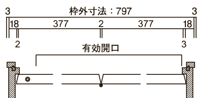
2枚扉 横断面図
