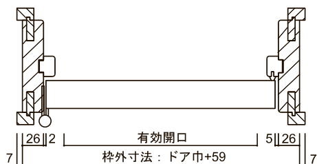
横断面図(親子ドア)
