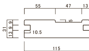
縦枠(片引用)
