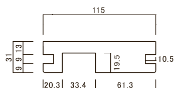
上枠(引違い用)
