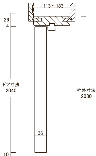
縦断面図
