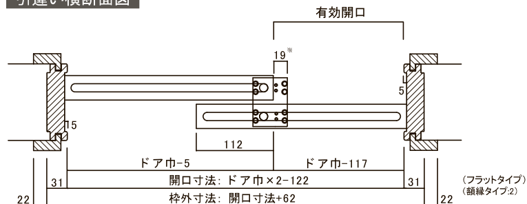
引違い横断面図
