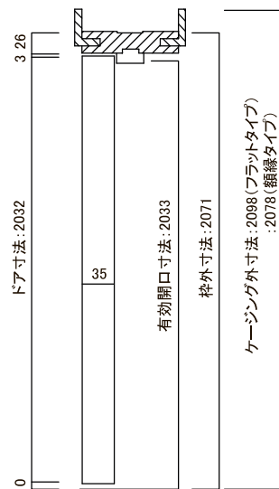
縦断面図
