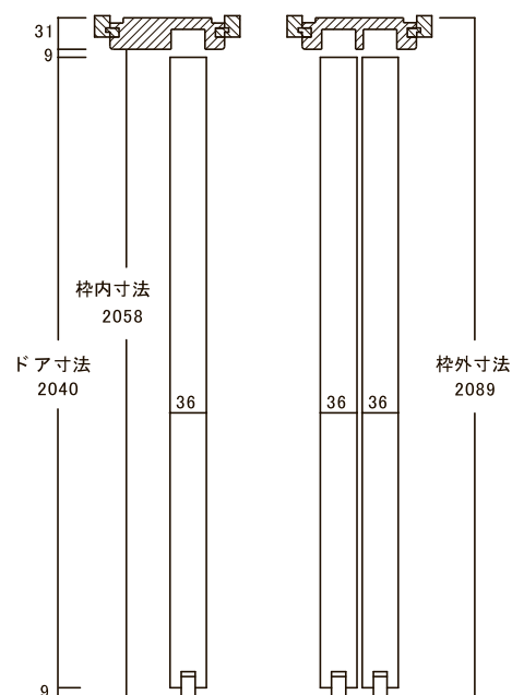
縦断面図
