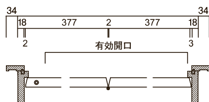
2枚扉 横断面図
