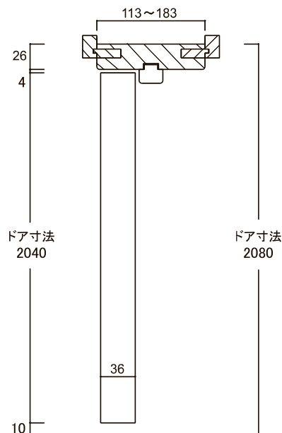
縦断面図
