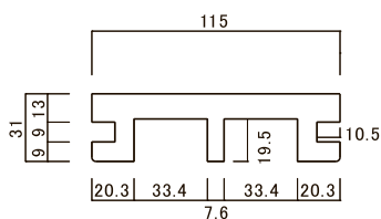
上枠(引違い用)
